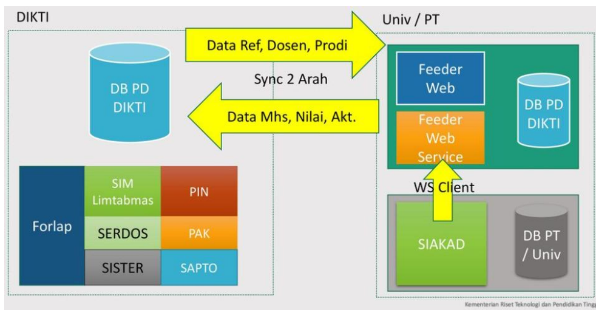
Gambar V.1 Arsitektur PD-Dikti
